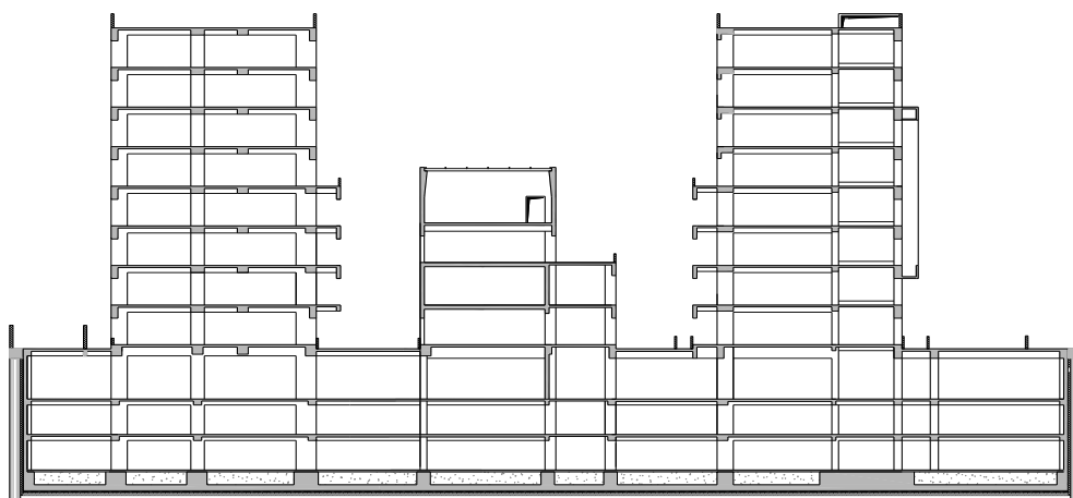
Τομή φέροντος οργανισμού
